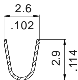
SEC. A-A
